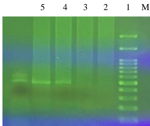
شکل ۲: شکل ژل الکتروفورز باکتری کلامیدوفیلا آورتوس با استفاده از نور فرابنفش، محصول مرحله اول PCR، M: bp DNA Ladder, Fermentas، نمونه‌های مثبت کلامیدوفیلا آورتوس در شیر: شماره ۴ و ۵، کنترل منفی کلامیدوفیلا آورتوس: شماره ۱، نمونه منفی کلامیدوفیلا آورتوس: شماره ۲، کنترل مثبت: شماره ۳
