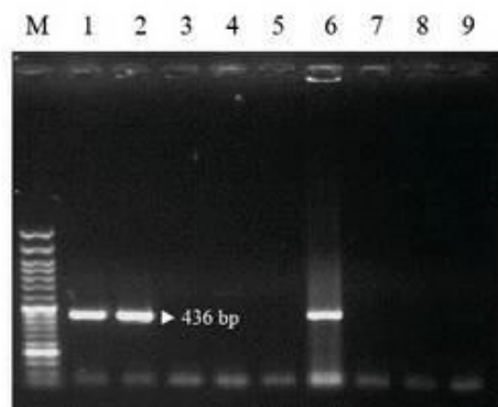
شکل ۱: شکل ژل الکتروفورز باکتری کلامیدوفیلا آورتوس با استفاده از نور فرابنفش، محصول مرحله اول PCR، M: bp DNA Ladder, Fermentas، نمونه‌های مثبت کلامیدوفیلا آورتوس در شیر: شماره ۱ و ۲، کنترل منفی کلامیدوفیلا آورتوس: شماره ۹، کنترل مثبت: شماره ۶
