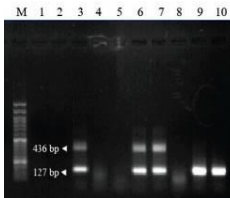
شکل ۳: شکل ژل الکتروفورز باکتری کلامیدوفیلا آورتوس با استفاده از نور فرابنفش، محصول مرحله دوم PCR، M: bp DNA Ladder, Fermentas، نمونه‌های مثبت کلامیدوفیلا آورتوس: شماره‌های ۳، ۶، ۷ و ۹، نمونه‌های منفی: شماره ۴ و ۵، کنترل مثبت کلامیدوفیلا آورتوس: شماره ۱۰
