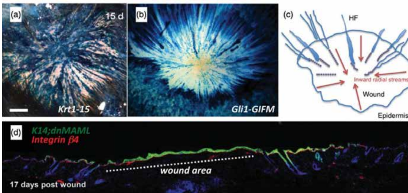
شکل ۳ - مشارکت نتایج سلولی مشتق از HF در اپیدرم زخم تازه ایجاد شده. جمعیت‌های مختلف سلول‌های مشتق از HF به‌صورت ژنتیکی ردیابی شده‌اند تا نقش سلول‌های مشتق شده از آن‌ها به بسته شدن زخم مشخص شود. (a) ردیابی موش‌های CrePR-15-Krt1 (که تقریباً ۷۰ درصد برآمدگی و ۵۰ درصد سلول‌های اپیدرمی غیربرآمده را قبل از زخم نشان می‌دادند) ۱۵ روز پس از آسیب، جریان‌های شعاعی نتایج سلولی مشتق از HF را نشان داد که به مرکز زخم هدایت می‌شدند. (b) تصویر مشابهی دو هفته پس از ایجاد زخم در موش‌های GIFM-Gli1 در فاز تلوژن مشاهده شد (c) این طرح شماتیک نشان می‌دهد که چگونه سلول‌های مشتق شده از HF به سمت داخل در جریان‌های شعاعی تکثیر می‌شوند. (d) جایگزینی کامل سلول‌های بدون برچسب در زخم (خط نقطه‌دار) با سلول‌هایی که dnMAML (نشاندار شده، سبز) ۱۷ روز پس از آسیب در موش‌های K14;dnMAML را بیان می‌کنند [۲۵].
