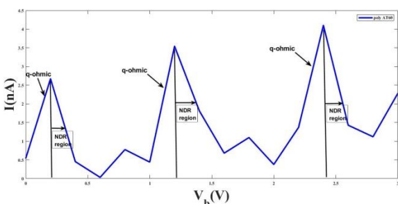
شکل ۲- نمودار مشخصه جریان-ولتاژ برای توالی AT - 60 bp
