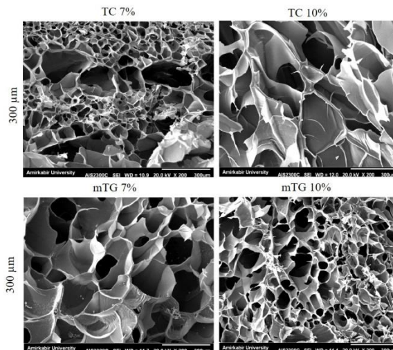
شکل ۳: تصاویر SEM هیدروژل تهیه شده با روش آنژیومی (mTG) و روش گرماسردی (TC) با غلظت‌های ۷ و ۱۰ درصد
