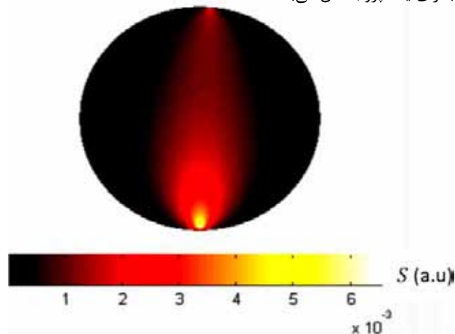
شکل ۲: تصویر یک ردیف از ماتریس ژاکوبین و حساسیت گره‌های مش
