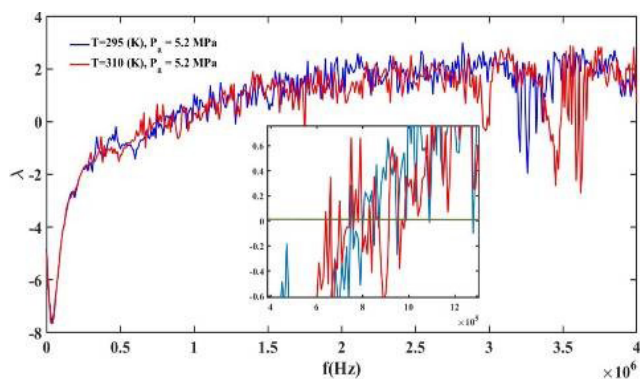
شکل ۴. نمودار لیاپانوف مربوط به فرکانس اکوستیک در فشار 5.2 MPa برای دو دما 295 K, 310 K
