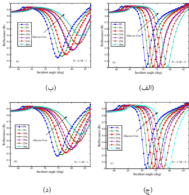
شکل 17- بازتاب با غلظت‌های مختلف گلوکز (الف) N = 0, M = 0 (ب) N = 0, M = 1 (ج) N = 1, M = 0 و (د) N = 1, M = 1 (ساختار پیشنهادی) [7].
