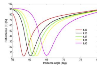
شکل 14- الف) ساختار زیست حسگر SPR برای تشخیص DNA (ب) نمودار بازتاب نسبت به ضریب شکست های مختلف DNA [45].
