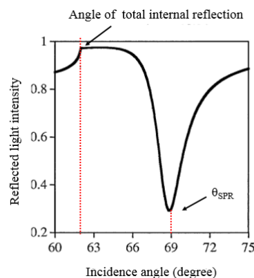
شکل 3- طیف بازتاب تابعی از زاویه نور فرودی در منشور برای تحریک پلاسmoniهای سطحی [48].
