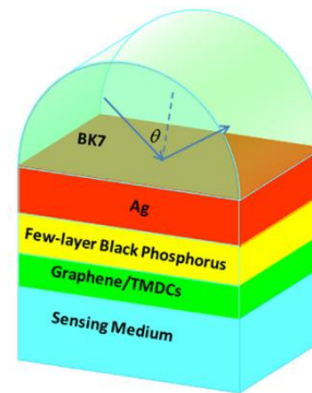
شکل 11- حسگر SPR متشکل از فسفر سیاه، گرافن و TMDCs [46].
