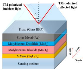
شکل 15- طرح واره زیست حسگر SPR پیشنهاد شده چندلایه برای تشخیص گلوکز [7].
