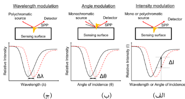
شکل 1- روش‌های مدولاسیون (الف) شدت (ب) زاویه‌ای (ج) طول موج [49].
