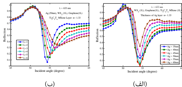
شکل 10- طیف بازتاب برحسب زاویه فرودی (الف) به ازای ضخامت‌های مختلف نقره
