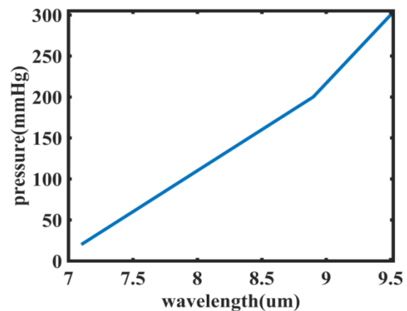
شکل-۱: نمودار فشار بر حسب طول موج تشدید
