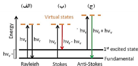
شکل ۱: نمودار سطوح انرژی در پراکنندگی طیف رامان. (الف): پراکنندگی رایلی، (ب): پراکنندگی استوکس رامان و (ج): پراکنندگی ضد استوکس رامان. h\nu انرژی نور ورودی و h\nu\nu انرژی نور ارتعاشی است [۱۵].
