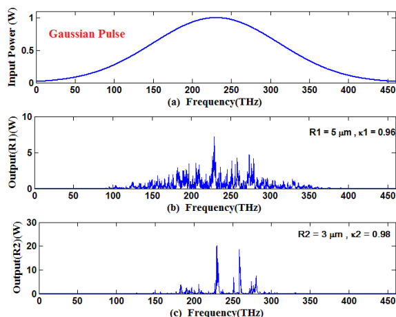
شکل ۲. نتایج حاصل از دو تشدیدکننده حلقه با طول موج مرکزی در ۱،۳ میکرومتر، جایی که (الف) پالس ورودی گاوسی، (ب) تولید سیگنال بی‌نظم، (ج) سیگنال‌های تقویت‌شده و فیلتر وجود دارد.
