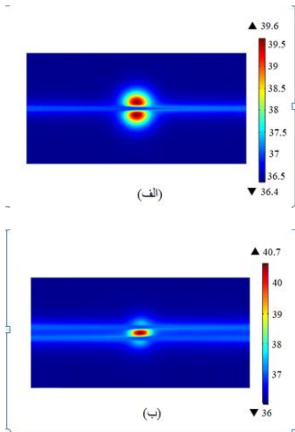
شکل ۶: توزیع دما در صفحه xy در هاپیترمیا به کمک لیزر با استفاده از نانوذرات با توزیع غیریکنواخت نانوذرات در تومور و مدت زمان انتشار ۳ ساعت، (الف) در عمق 4/2 \text{ mm} و در حضور یک رگ (ب) در عمق 2/5 \text{ mm} و در حضور دو رگ
