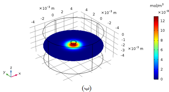
شکل: توزیع نانوذرات در ناحیه توموری در صفحه xy عبوری از مرکز تومور پس از الف) ۰/۵ ساعت انتشار، ب) ۱ ساعت انتشار، ج) ۲ ساعت انتشار، د) ۳ ساعت انتشار و ه) ۴ ساعت انتشار نانوذرات
