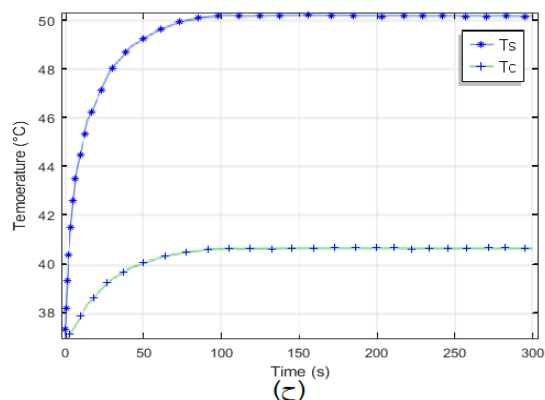
شکل ۷: توزیع دما در هاپیترمیا به کمک لیزر با استفاده از نانوذرات با (الف) و (ب) توزیع یکنواخت، (ج) و (د) توزیع غیریکنواخت در تومور و مدت زمان انتشار ۳ ساعت، (ه) و (و) توزیع غیریکنواخت و مدت زمان انتشار ۳ ساعت و در حضور یک رگ، (ز) و (ح) توزیع غیریکنواخت و مدت زمان انتشار ۳ ساعت و در حضور دو رگ
