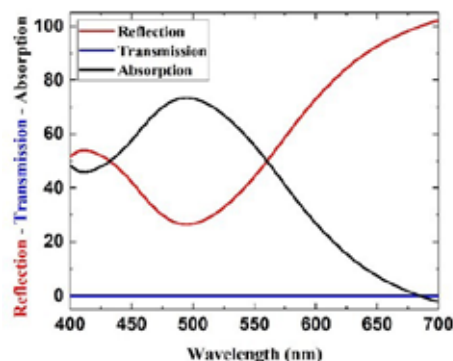
شکل ۳: طیف جذب، بازتاب و عبور ابرجاذب
