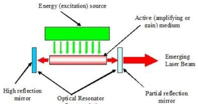
شکل ۱: اجزای یک سیستم تولید لیزر شامل سیستم پمپ اپتیکی مارپیچ در لیزر یاقوت
