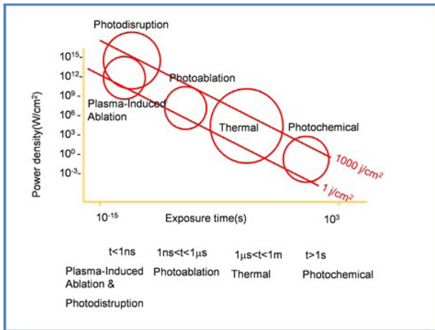
شکل ۴: نمودار مکانیسم‌های برهمکنش لیزر - بافت
