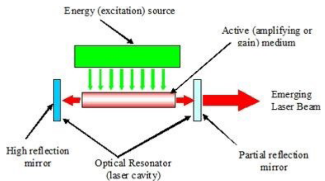
شکل ۱: اجزای یک سیستم تولید لیزر شامل سیستم پمپ اپتیکی ماریچ در لیزر یاقوت
