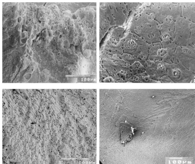
شکل ۶: ایجاد ذوب‌شدگی در عاج دندان با استفاده از لیزر Nd:YAG [۲]
