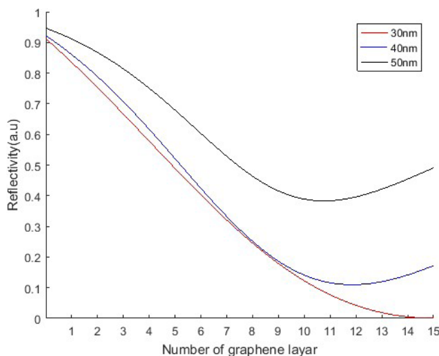
شکل ۸: نمودار تغییرات حداقل بازتاب برحسب تعداد لایه‌های گرافن برای نقره در بهینه زاویه تشدید برای ضخامت‌های متفاوت لایه فلزی در طول موج ۶۳۲/۸ نانومتر
