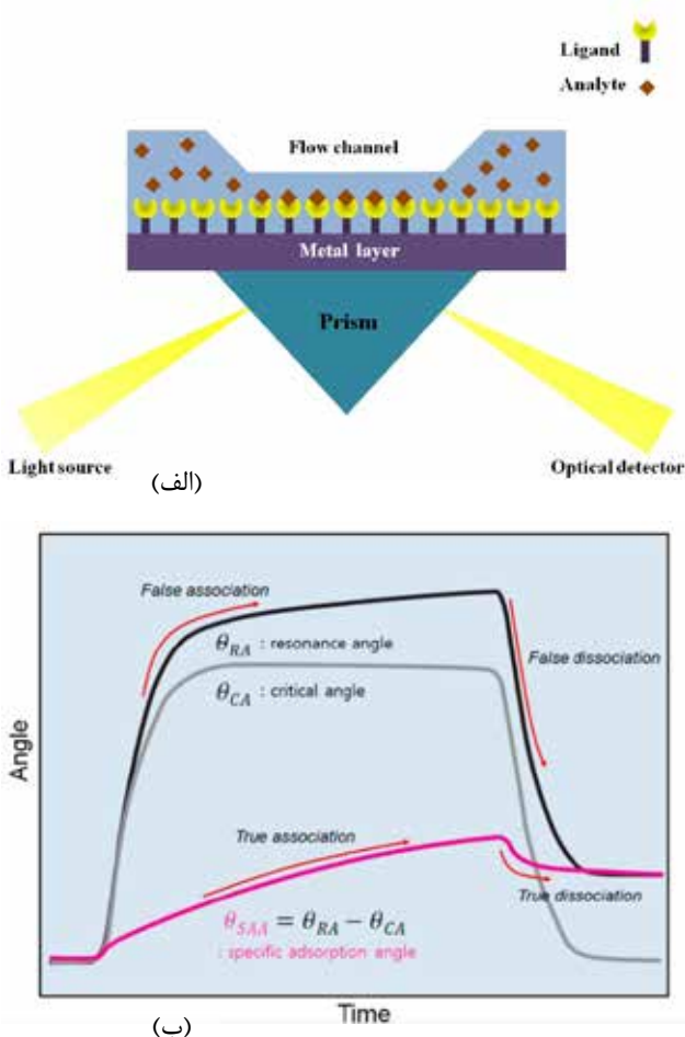
شکل ۱: ساختار حسگرهای SPR شامل گیرنده‌های ثابت زیستی و شیمیایی (لیگاند) و نمونهٔ مورد بررسی (آنالایت) (الف). نمودار بررسی عملکرد حساسیت‌سنجی بیوسنسرهای مبتنی بر تشدید پلاسمون سطحی (ب)
