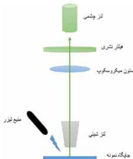
شکل ۷: جایگاه منبع لیزر در زاویه ۴۵ درجه روی سکوی نمونه و موقعیت سایر قطعات اپتیکی میکروسکوپ
