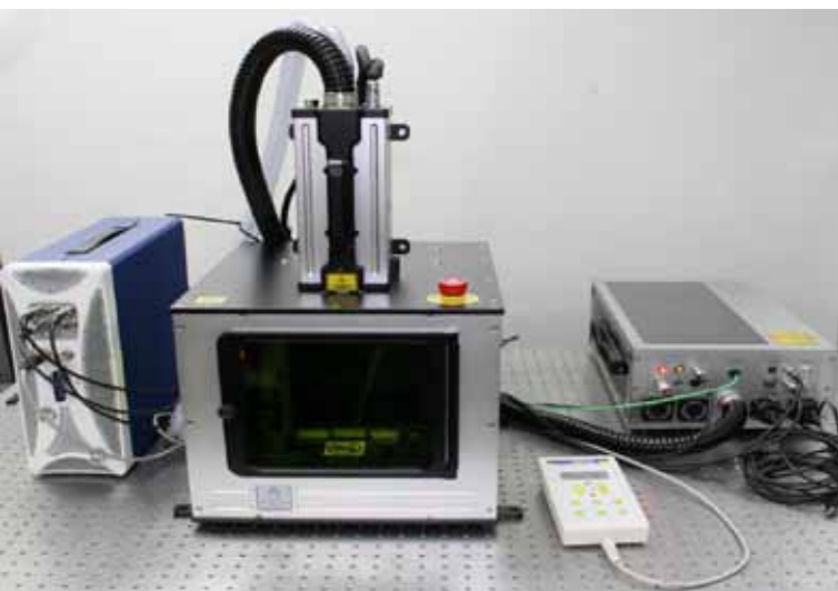
شکل ۲: سامانه LIBSCAN ۱۰۰۰
