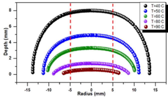
شکل ۴: نمودار کانترهای دمایی در ناحیه تومور و بافت سالم در زمان تابش ۱۱۰ s، شدت تابش 1 W/cm 2 و نانومیل‌های طلا با غلظت ۰/۰۰۱ درصد
