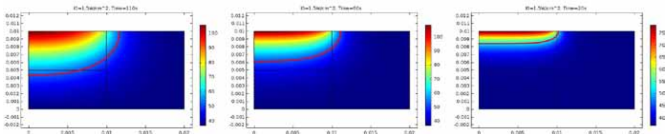
شکل ۷: الف) توزیع دما در ناحیه تومور و بافت سالم در شدت تابشی 1/5 \text{ W/cm}^2 و زمان‌های پرتودهی ۱۰، ۲۰ و ۳۰ ثانیه. خط قرمز مشخص‌کننده مرز کسر تخریب حرارتی کامل ( \Omega=1 ) است که در ناحیه بالای آن \Omega \geq 1 و در ناحیه پایین آن \Omega \leq 1 است.
