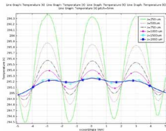
شکل ۴: تغییرات دما در راستای محور x به‌ازای عمق‌های مختلف از بافت z و p=3 mm برای پرتوی ورودی سر تخت
