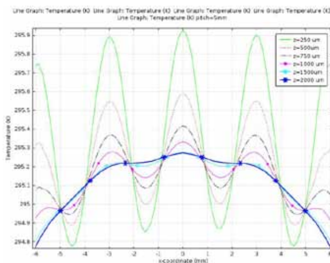
شکل ۶: تغییرات دما در راستای محور X به‌ازای عمق‌های مختلف از بافت Z و p=۳mm برای پرتوی ورودی گاوسی
