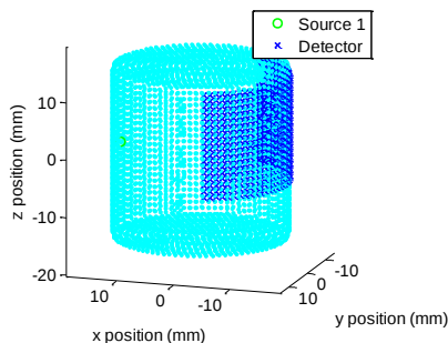
شکل ۲: نمای ۳د بعدی از موقعیت نسبی لیزر و آشکارساز در یک پروجکشن
