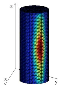
شکل ۶: شدت رسیده به سطح پس از اعمال تقریب بورت
