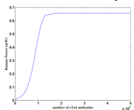
شکل ۶: تغییرات توان سیگنال رامان خروجی لیزر بر حسب غلظت cTnI
