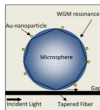
شکل ۴: نمایی از حسگر میکروکره-فیبر نوری با نانو ذرات طلا برای آشکارسازی cTnI
