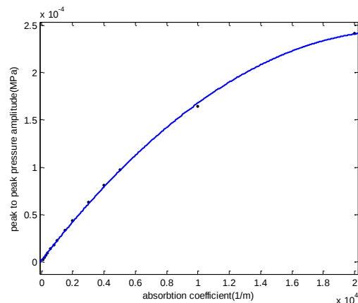
شکل ۱۱: دامنه موج اکوستیک در مقابل ضریب جذب تومور در محدوده وسیعی از ضریب جذب
