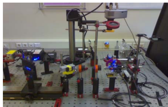
شکل ۲: چیدمان اپتیکی
