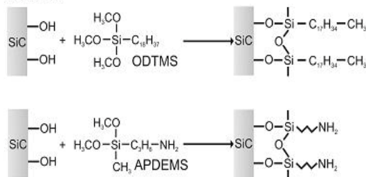
شکل ۴: فرآیند سایلیزاسیون
