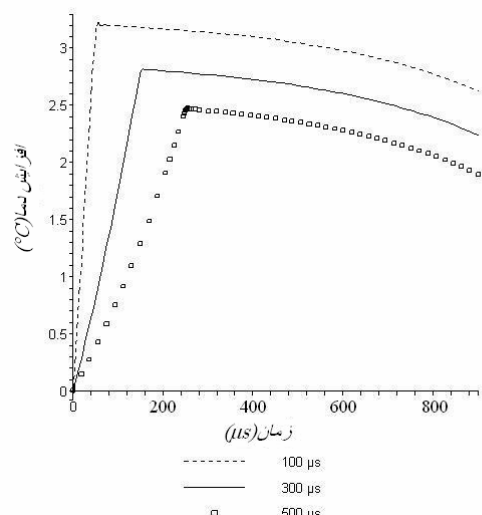
شکل ۲- نمودار تغییرات زمانی اختلاف دما، برای سه مدت زمان پالس مختلف و با انرژی پالس ۳۰۰ mJ
