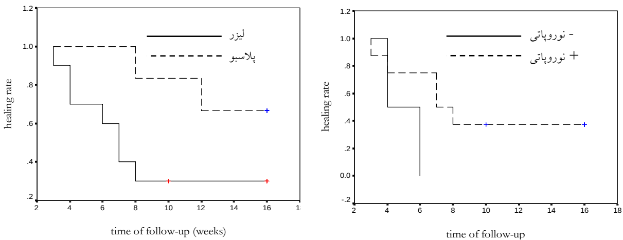
شکل ۱- منحنی بقای Kaplan-Meier برای بیمارانی که تحت درمان لیزر روشن و لیزر خاموش (پلاسیبو) قرار گرفتند (سمت چپ). میزان بهبودی ۱۶ هفته بیمار پس از لیزر درمانی ۷۰٪ در مقایسه با گروه پلاسیبو ۳۳٪ بود. p = ۰/۰۷۲ (آزمون Log-rank). منحنی بقای Kaplan-Meier در بیمارانی که تحت درمان لیزر روشن در دو گروه وجود یا عدم وجود نوروپاتی (سمت راست). زمان متوسط برای بهبودی کامل زخم در گروه بدون نوروپاتی ۷ \pm ۱/۸۹ هفته با حدود اطمینان ۹۵٪ برابر با ۳/۳-۱۰/۷ هفته می باشد. p = ۰/۱۱۲ (آزمون Log-rank).
