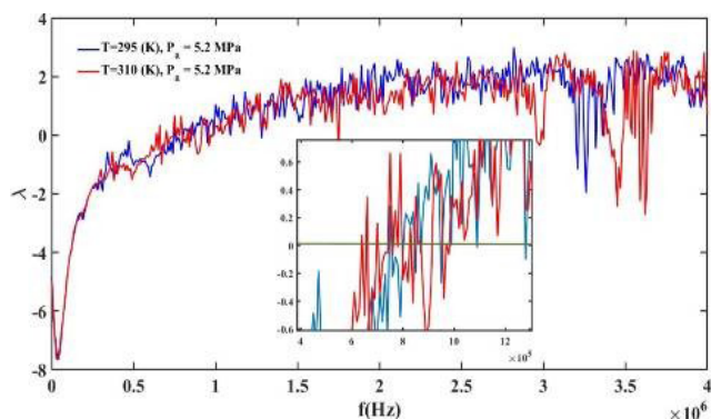
شکل ۴. نمودار لیپانوف مربوط به فرکانس آکوستیک در فشار 5.2 MPa برای دو دما 295 K, 310 K
