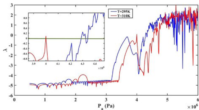
شکل ۳. نمودار مربوط به فشار اکوستیک در دماهای مختلف با فرکانس یکسان 3.2 MHz
