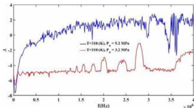
شکل ۵. نمودار لیپانوف مربوط به فرکانس اکوستیک در دمای یکسان 310 K در فشارهای متفاوت
