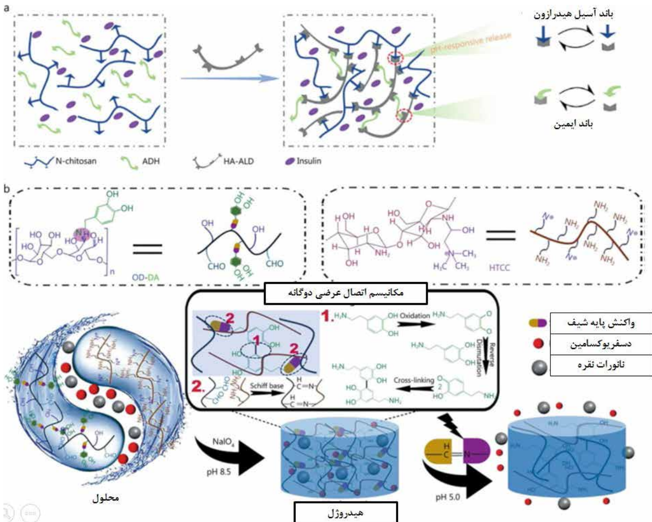
شکل ۵. فرآیند ساخت و ساختار هیدروژل‌های نمونه پاسخگو به pH (الف) سنتز هیدروژل‌های پاسخگو به pH حاوی انسولین براساس پیوندهای آسیدل هیدرازون [۲۸]. (ب) مکانیسم سنتز هیدروژل پاسخگو به pH براساس پیوند باز شیف دوگانه و نمودار شماتیک فرآیند آزادسازی AgNPs و دفریکسامین در شرایط اسیدی. دی‌هیدرازید اسید آدیپیک ADH، نانوذرات نقره AgNPs، اسید هیالورونیک-آلدئید HA-ALD، N-کیتوزان-کربوکسیل اتیل کیتوزان، OD-DA اکسیدشده دکستران-دوپامین، کیتوزان HTCC نمک آمونیوم چهارتایی
