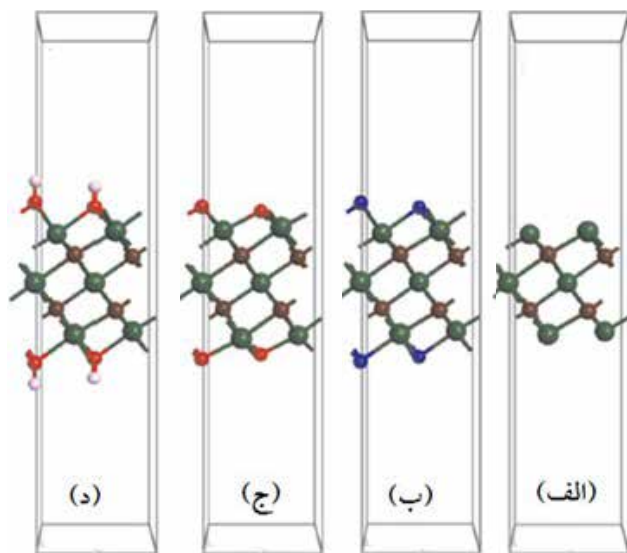
شکل ۲- ساختار بلوری MXene Ti_3C_2T_x (الف) Ti_3C_2F_x (ب) Ti_3C_2O_x (ج) Ti_3C_2(OH)_x (د) [۲]
