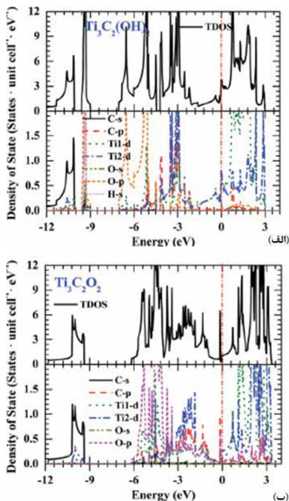
شکل ۶- چگالی حالت‌ها برای (الف) \text{Ti}_3\text{C}_2(\text{OH})_2 MXene و (ب) \text{Ti}_3\text{C}_2\text{O}_2 MXene [۱۷].
