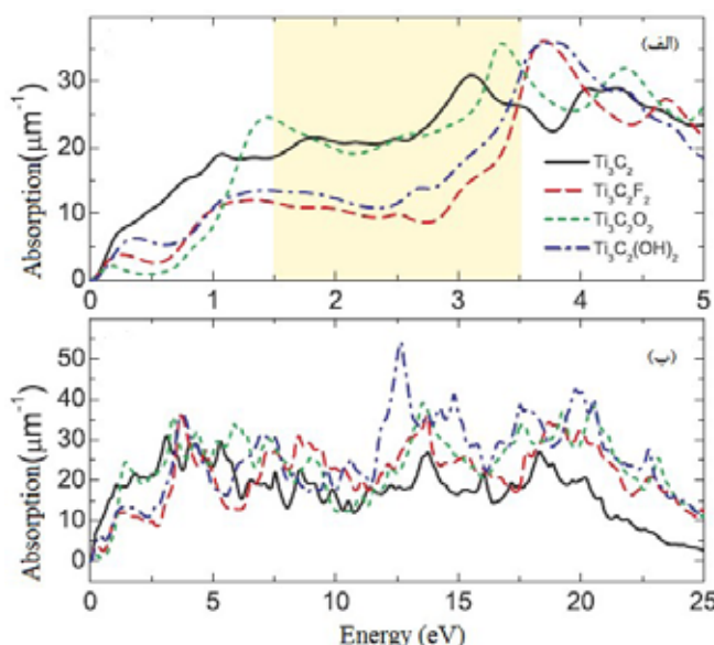
شکل ۱۱- نمودار طیف جذب برای \text{Ti}_3\text{C}_2\text{ MXene} و پایانه‌های سطحی مختلف [۲]
