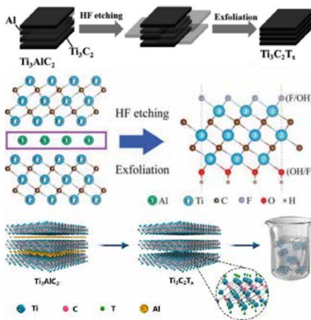
شکل ۳- تولید Ti_3C_2T_x از پیش‌ماده Ti_3AlC_2 [۱۷]
