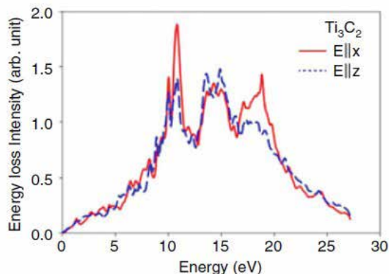
شکل ۹- (الف) نمودار بخش حقیقی و موهومی تابع دی‌الکتریک (ب) طیف بازتاب (ج) طیف جذب (د) طیف اتلاف انرژی برای قطبش میدان الکتریکی موازی ( E||x ) و عمود ( E||z ) از \text{Ti}_3\text{C}_2 \text{MXene} [۶، ۱۲]
