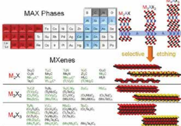
شکل ۱. طرحواره ساختاری مکس فازها با رابطه عمومی M_{n+1}AX_n و مکسین ها با رابطه عمومی M_{n+1}X_nT_x
