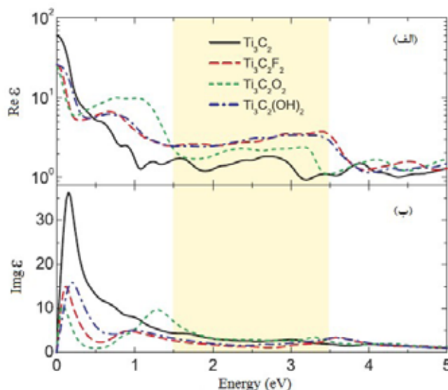
شکل ۱۰- نمودار بخش حقیقی و موهومی تابع دی‌الکتریک وابسته به فرکانس، برای \text{Ti}_3\text{C}_2\text{ MXene} و گروه‌های سطحی مختلف [۲]
