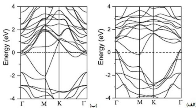
شکل ۵- ساختار نوار انرژی \text{Ti}_3\text{C}_2\text{O}_2 (الف) و \text{Ti}_3\text{C}_2(\text{OH})_2 (ب) [۱۷]
