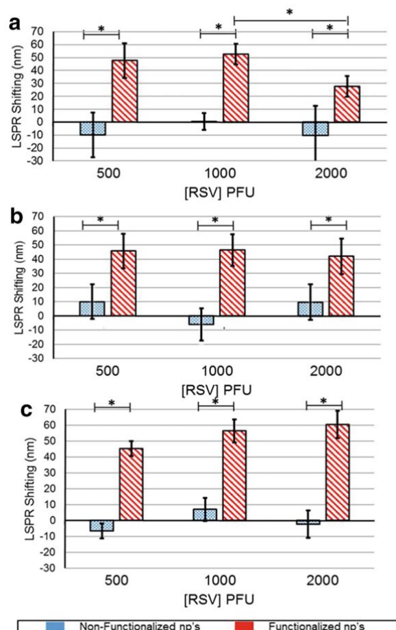
شکل 5- نمودار شیف رزونانس پلاسمون سطحی موضعی را در تیرهای مختلف ویروس سنسیشیال تنفسی در 30 دقیقه (a)، 60 دقیقه (b) و 120 دقیقه (c) برای نانوذرات نقره دارای آنتی بادی عملکردی (قرمز) و غیر عملکردی (آبی) نشان می دهد. نماد ستاره نشان دهنده معنی داری p < 0.05 است [83].
