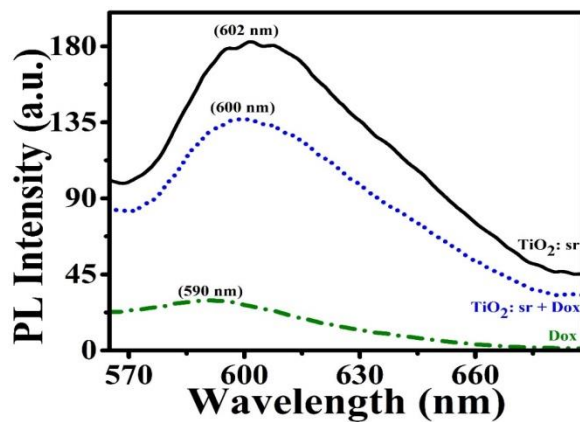
شکل ۳: طیف فوتولومینسانس (PL) نانوذرات TiO 2 :Sr و Dox و TiO 2 که با طول‌موج ۴۵۰ نانومتر تحریک شده‌اند.
