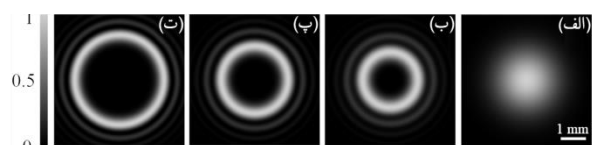
شکل ۲: توزیع شدت (الف) باریکه گاوسی و باریکه های چرخان با بار توپولوژیک (ب) ۲، (ج) ۴ و (د) ۷.
