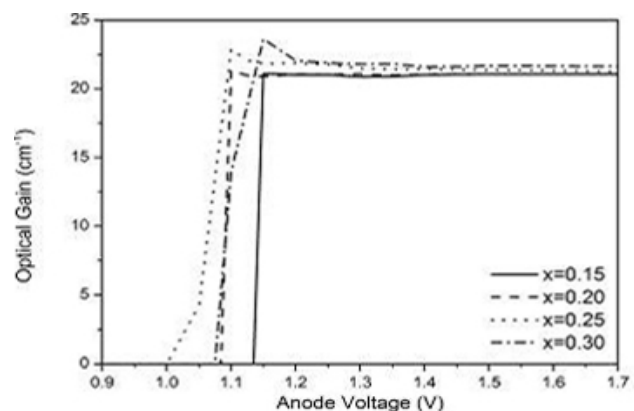
شکل ۹: تغییرات بهره اپتیکی برحسب ولتاژ بایاس به ازای مقادیر گوناگون x
