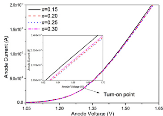
شکل ۸: مشخصه جریان-ولتاژ لیزر گسیلنده جانبی فابری-پرو \text{In}_x\text{Ga}_{1-x}\text{AsP} به ازای مقادیر گوناگون x . داخل شکل نمودار با مقیاس بزرگ‌تر نشان داده شده است.
