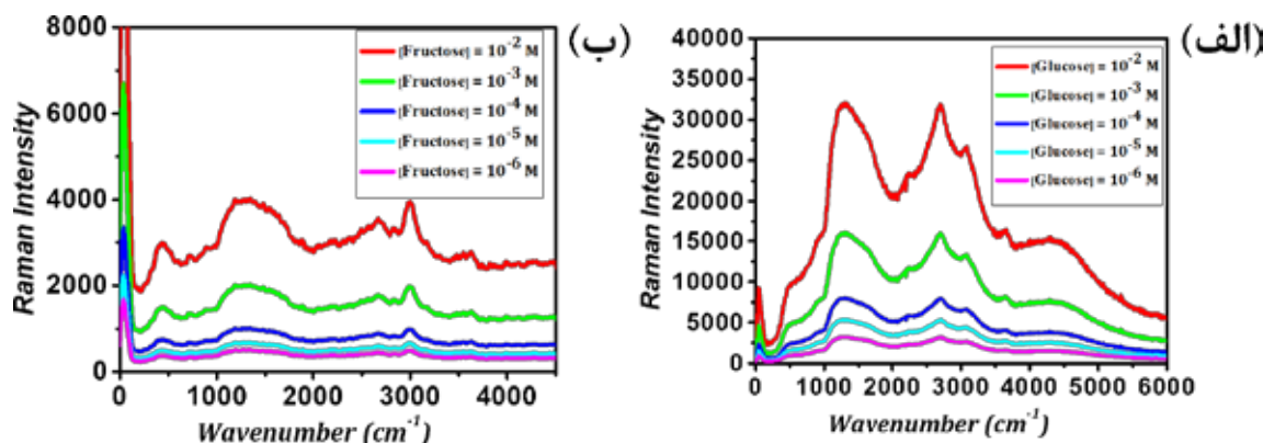
شکل ۶: طیف SERS (الف) گلوکز و (ب) فروکتوز با غلظت‌های ۱۰ -۲ ، ۱۰ -۳ ، ۱۰ -۴ ، ۱۰ -۵ و ۱۰ -۶ مولار حکاکی‌شده بر روی بستر پلاسمونیک
