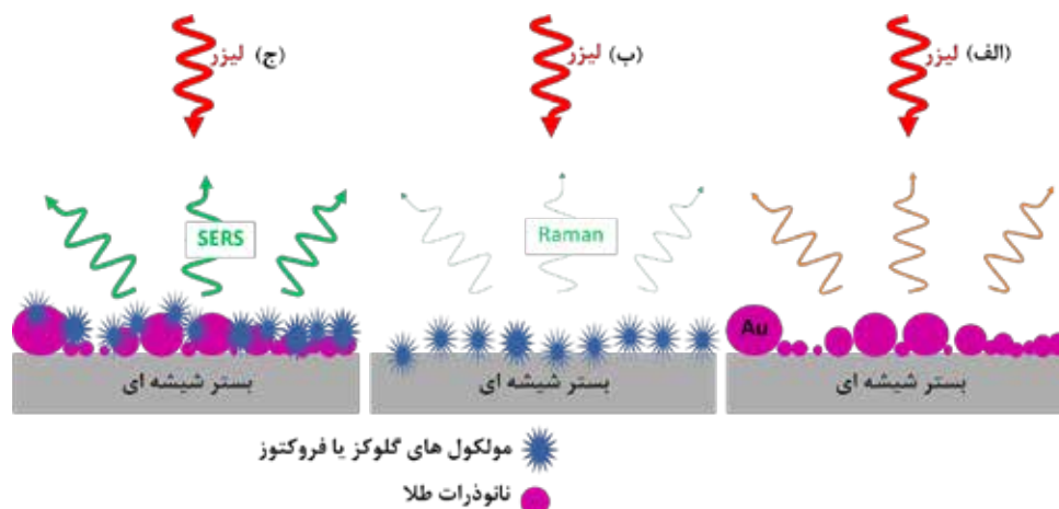
شکل ۱: طرحواره آشکارسازی و مشاهده الف) سیگنال رامان حاصل از بستر پلاسمونیک، ب) سیگنال رامان حاصل از مولکول های گلوکز یا فروکتوز حکاکی شده روی زیرلایه شیشه ای، ج) سیگنال SERS مولکول های گلوکز و فروکتوز حکاکی شده روی بستر پلاسمونیک که بهبود سیگنال رامان مولکول های گلوکز و فروکتوز حکاکی شده روی بستر پلاسمونیک نسبت به سیگنال رامان مولکول های گلوکز یا فروکتوز که در معرض تشدید پلاسمون های سطحی نانوذرات طلا قرار نگرفته است را نمایش می دهد.
