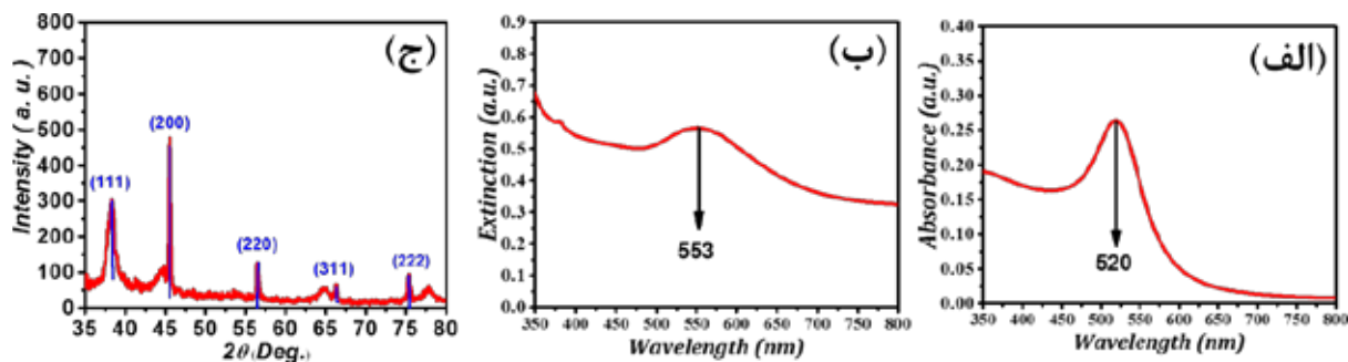
شکل ۲: الف) طیف جذب نانوذرات طلا ساخته‌شده به روش شیمیایی با عامل کاهنده تری‌سدیم سیترات دوا به با بیشینه جذب در طول موج ۵۲۰ نانومتر، ب) طیف خاموشی بستر پلاسمونیک با بیشینه جذب در طول موج ۵۵۳ نانومتر و ج) الگوی پراش اشعه ایکس نانوذرات طلا
