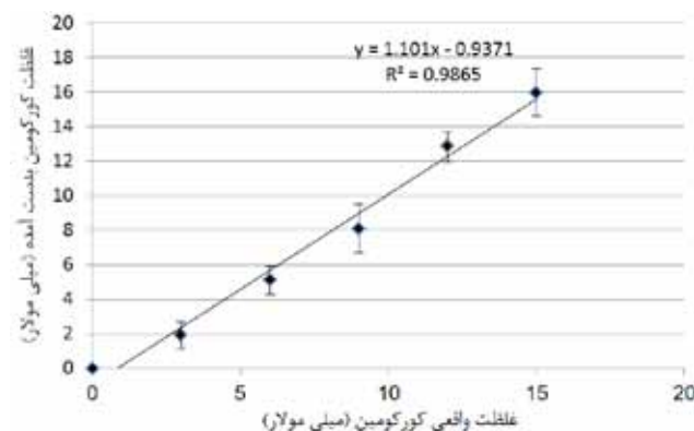
شکل ۴: نمودار مقایسه غلظت واقعی نانوکورکومین با غلظت به دست آمده از برازش بیناب بازتاب تجربی و تئوری
