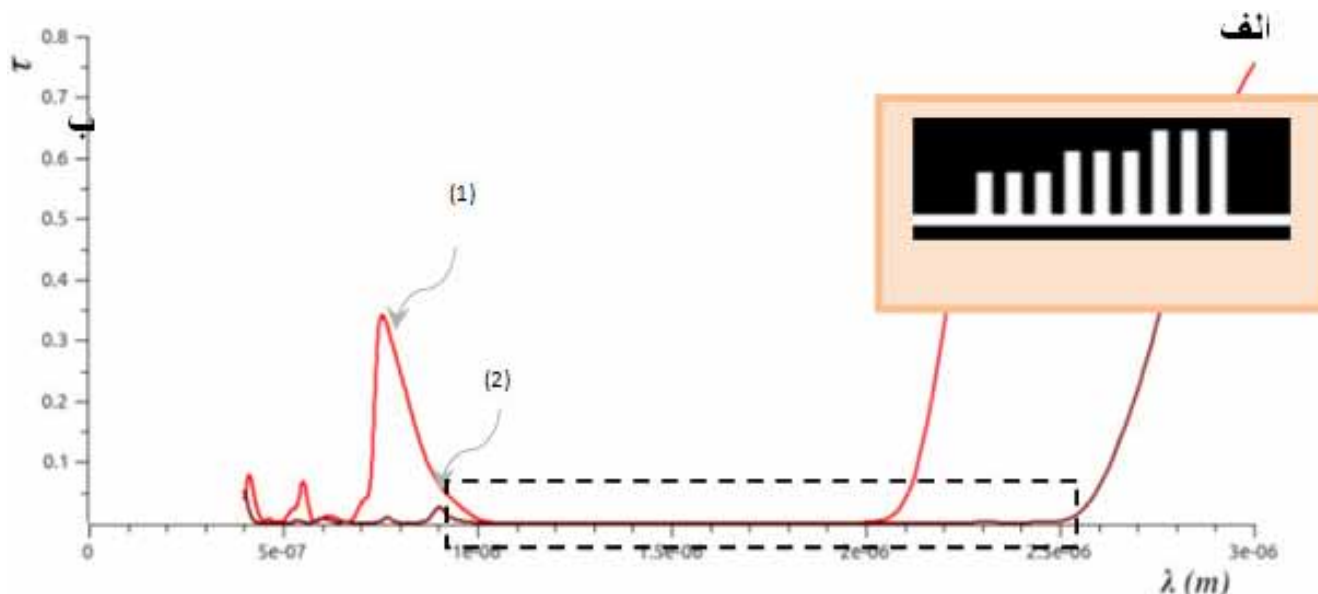
شکل ۳: الف) مقطع عرضی از C3-3-TPNF (ب) بیناب‌های گذردهی نسبی C3-3-TPNF بیناب (۱) و C3-3-3-TPNF بیناب (۲)
