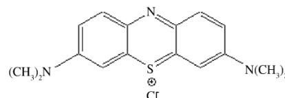
شکل ۱: ساختار مولکولی متیلن‌بلو [۱۲]
