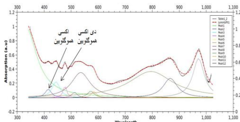
شکل ۴: طیف گرفته‌شده از لب شخصی که دارای رنگ لب تیره می‌باشد. محل پیک‌های اکسی‌هموگلوبین و دی‌اکسی‌هموگلوبین با پیکان نشان داده شده‌است. نسبت دی‌اکسی‌هموگلوبین به اکسی‌هموگلوبین تعیین‌کننده تیرگی لب افراد است.
