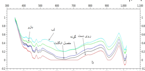
شکل ۳: مقایسه طیف‌های گرفته‌شده از نواحی مختلف پوست. هرچه میزان خون در آن ناحیه بیشتر و در نتیجه پوست سرخ‌تر بوده، طیف آن ناحیه در بالاتر قرار گرفته‌است.
