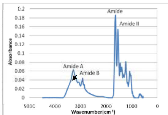
شکل ۳: طیف مادون قرمز بافت کپسول قبل از تابش فرابنفش
