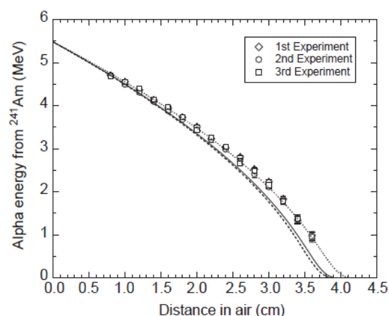
شکل ۴- نمودار انرژی ذرات آلفای چشمه ^{241}\text{Am} با انرژی اولیه 5.5\text{ MeV} بصورت تابعی از مسافت طی شده با استفاده از معادله (6) و معادله (7) ۱۵ پارامتری
